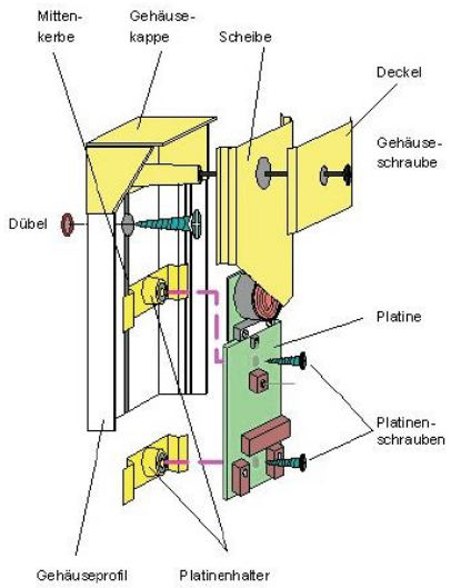
Bild 10: Wandmontage
