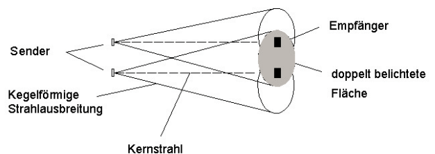
Bild 4: Doppelbelichtung am Empfänger
