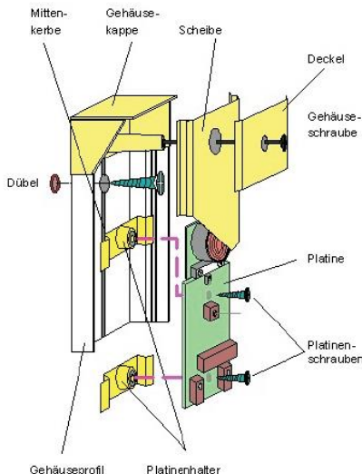
Bild 10: Wandmontage
