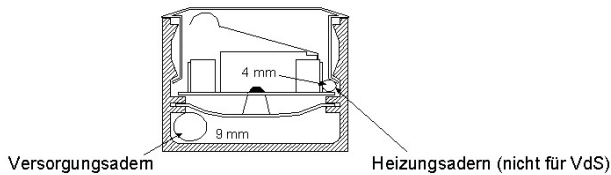
Bild 9: Kabelführung
