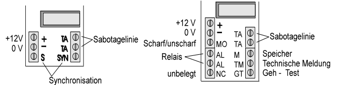
Bild 13: Verdrahtungsschema für Mehrkanalbetrieb
